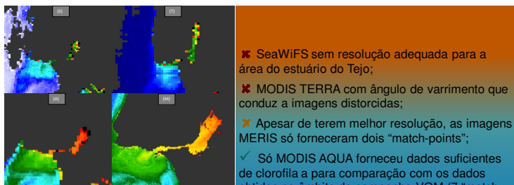
Fig. 2: Imagens de concentração de clorofila a, no estuário do Tejo, obtidas através dos diferentes sensores no dia 26 de Setembro de 2006: SeaWiFS (S); Modis Terra (T); Modis Aqua (A); e Meris (M). Imagens processadas no BEAM VISAT (Brockmann Consult). Área de estudo (WGS 84, decimal): 38.9613N a 38.5690N e 9.5108W a 8.8079W.
