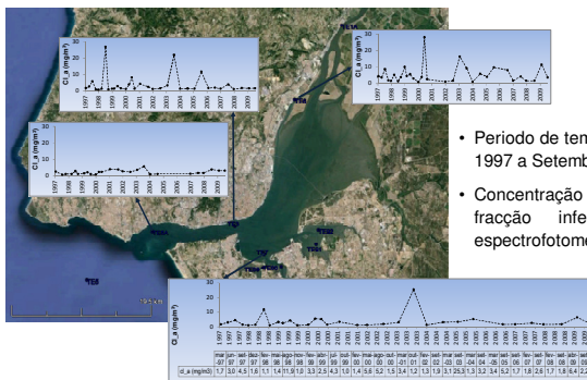
Fig. 1. Séries temporais de clorofila a (Cl_a) em mg/m³, determinadas para alguns pontos de amostragem do estuário do Tejo, durante o período de Março de 1997 a Setembro de 2009 (representado em abcissas). Na série correspondente ao ponto TE7 também está representada a tabela de dados para visualização dos dias de amostragem (Fonte da imagem: Google Earth).
