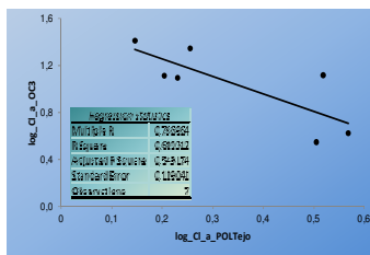
Fig. 3: Correlação entre logaritmos dos dados de clorofila a obtidos pelo POLTejo ( \log_{Cl_a\_POLTejo} ) e MODIS AQUA ( \log_{Cl_a\_OC3} ).
