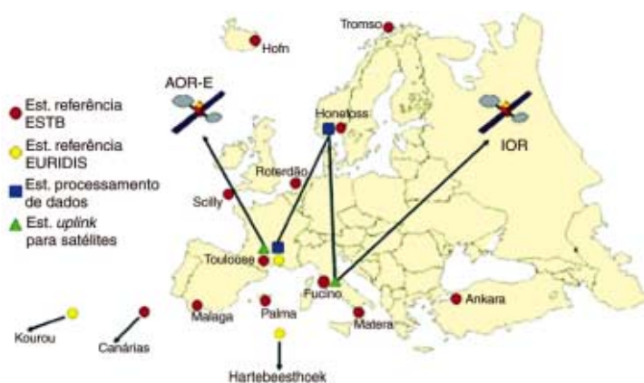
Arquitectura do EGNOS na sua fase pré-operacional
