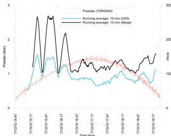
Figura 3. Registo de 10 em 10 min. da Moda e D50 ( \mu\text{m} ). A linha a vermelho representa a altura de água (pressão dbar).
