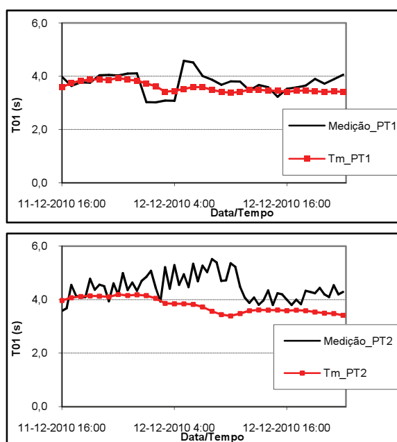
Fig. 4 – Períodos T_{01} em PT1 (cima) e PT2 (baixo), 11 e 12 de Dezembro.
