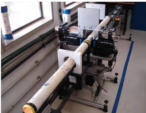
Fig. 2: Multi - Sensor Core Logger (MSCL) da GEOTEK.
