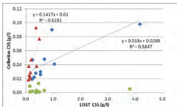
Figura 7. Correlação linear entre CSS obtida pelo LISST e pelas colheitas com garrafas (a azul-CSS total; a verde-CSS >63µm e a vermelho <63µm).
