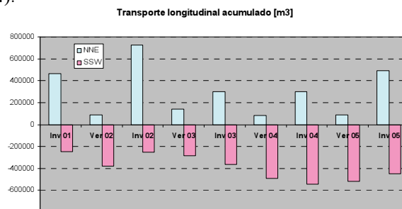
Fig. 3. Transporte longitudinal sazonal num perfil transversal central
