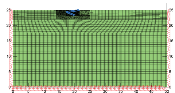
Fig. 6. Visão geral do modelo FEM utilizado.
