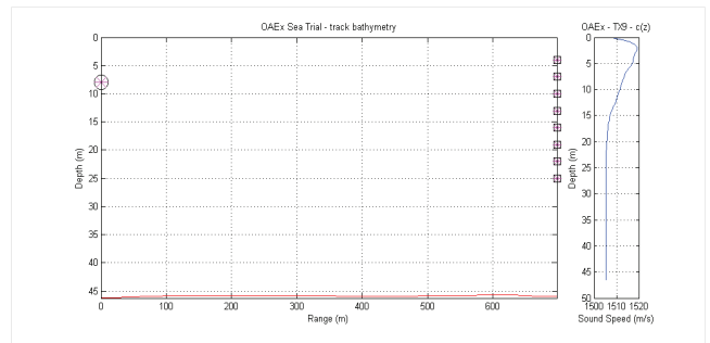
Fig.4: TX9. Perfis batimétrico e de velocidade do som com a geometria dos transdutores no experimento OAE' 10
