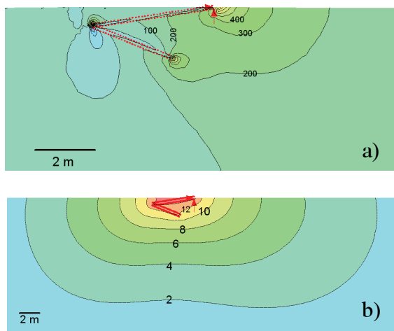
Fig. 7. Gráficos pela análise de FEM: a) tensões máximas no solo em kPa; b) deslocamentos máximos na horizontal em centímetros.
